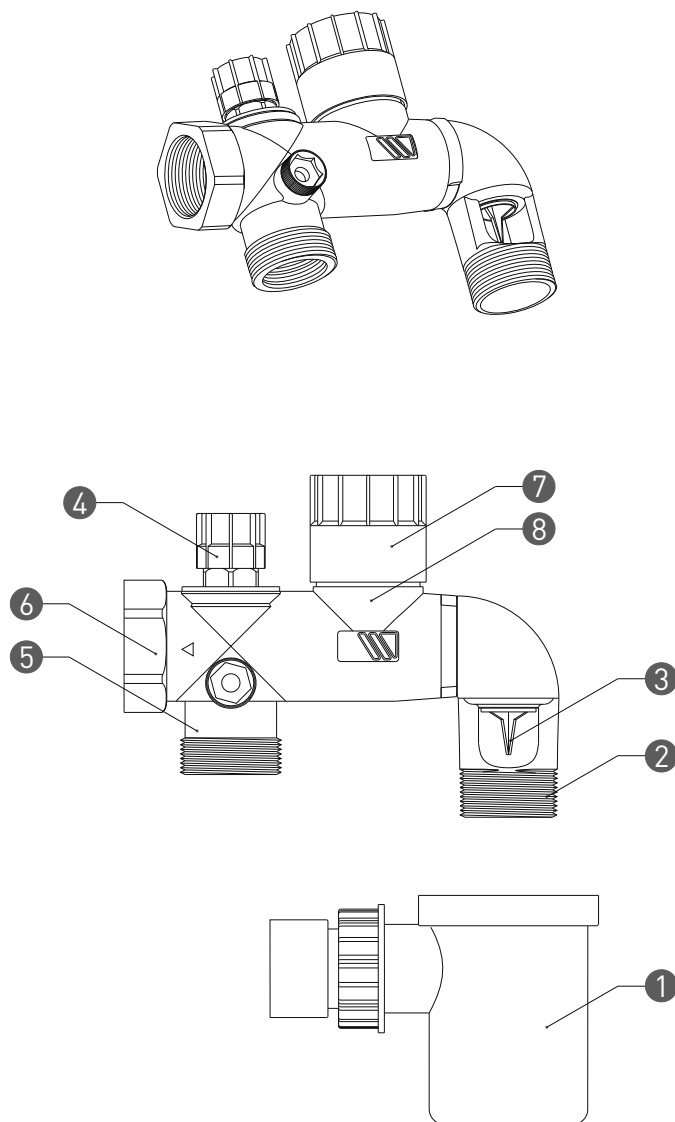
Fig. 4 - Grupo Hidráulico 1"
