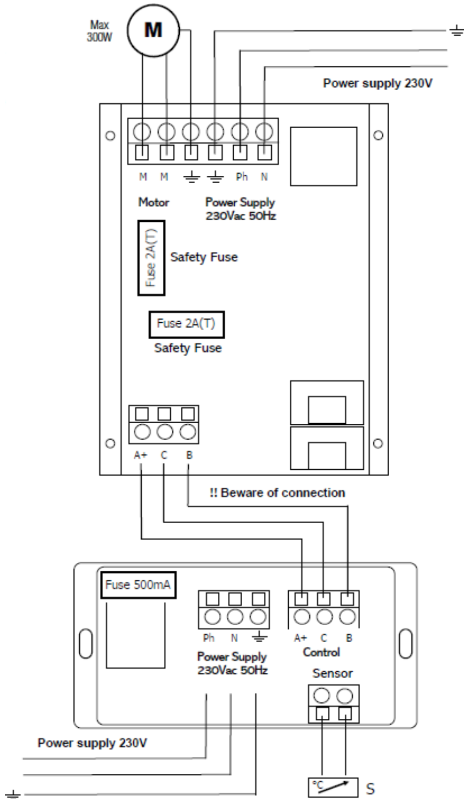
Figura nº12 - Conexões a serem feitas no controlador e no módulo de potência do Itaca eco C / V
