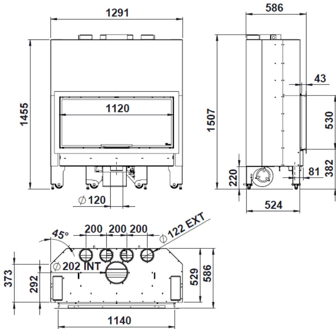
Figura nº3 - Dimensões em mm do aparelho ITACA 120 eco
