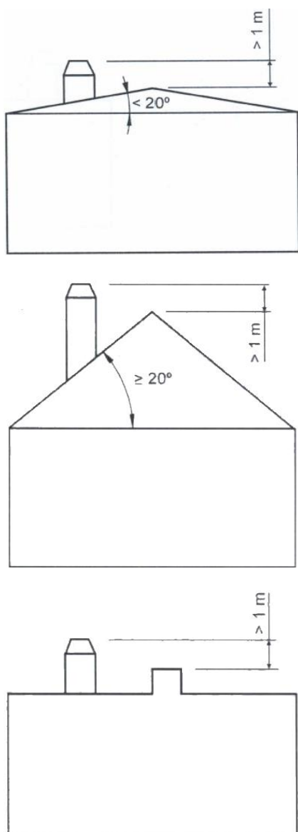
Figura nº22 - Distâncias desde o acabamento até à cumeeira do telhado
