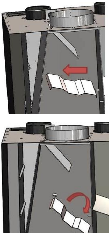
Figura nº33 - Desmontagem do defletor superior Itaca 80
