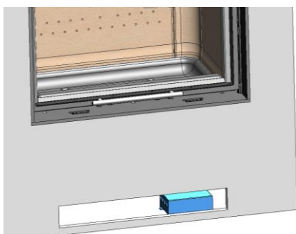
Figura n°19 - Posicionamento do módulo de potência em frente à grade de ventilação frontal
