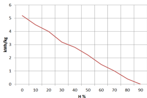
Figura n°25 - Relação entre humidade e poder calorífico da lenha.
