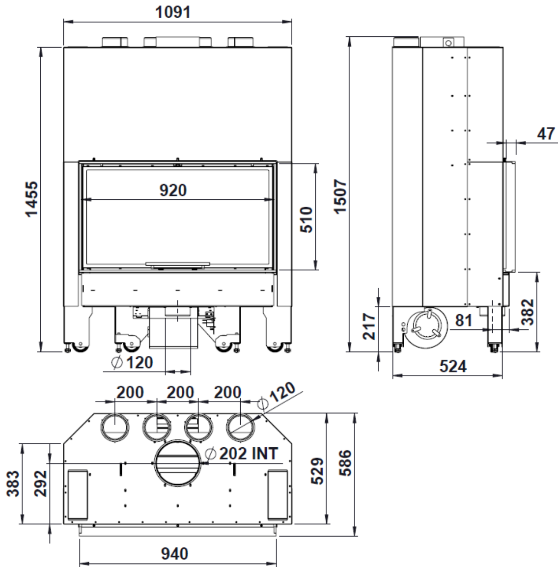
Figura nº2 - Dimensões em mm do aparelho ITACA 100 eco
