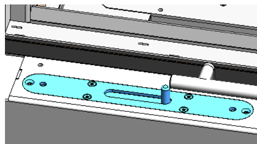
Figura nº49 - Registos removíveis
