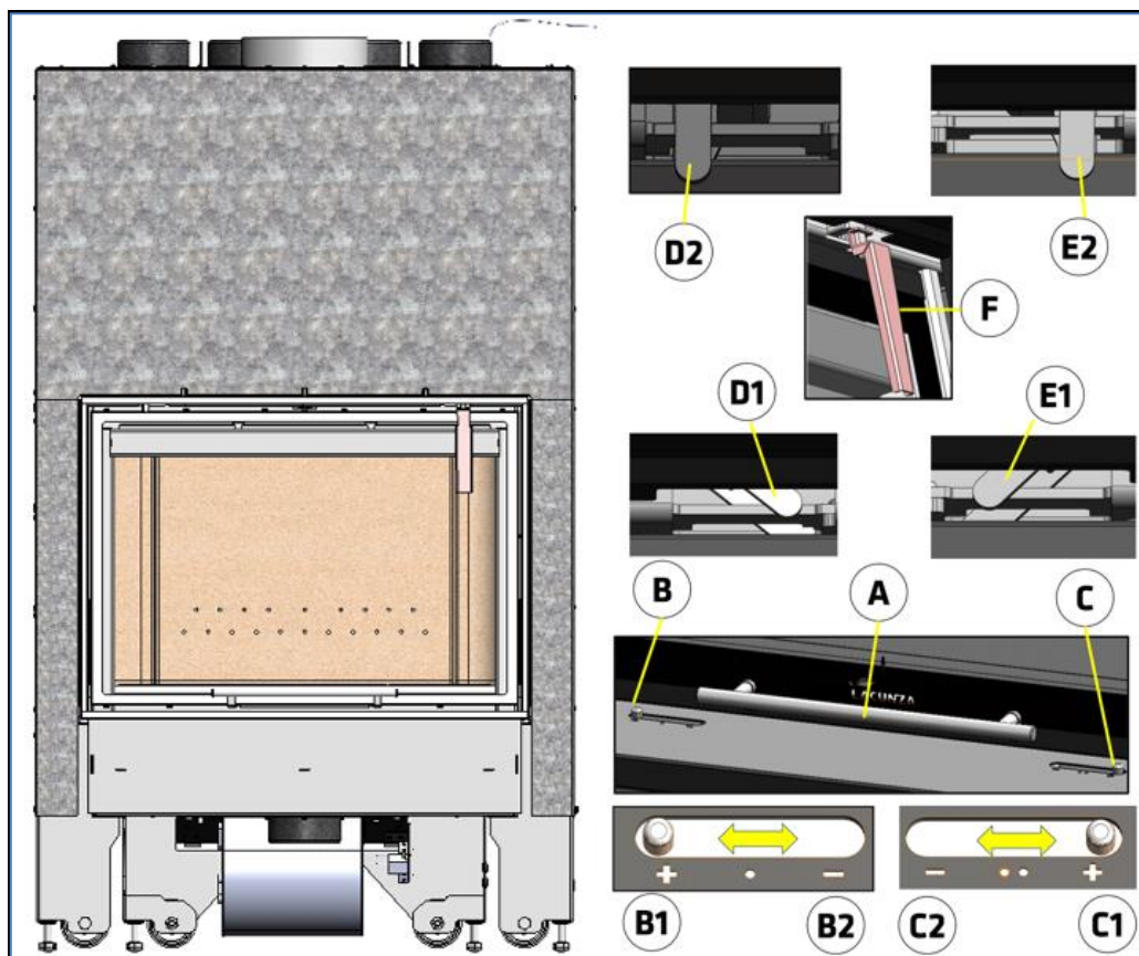
Figura n°26 - Elementos de funcionamento do aparelho
