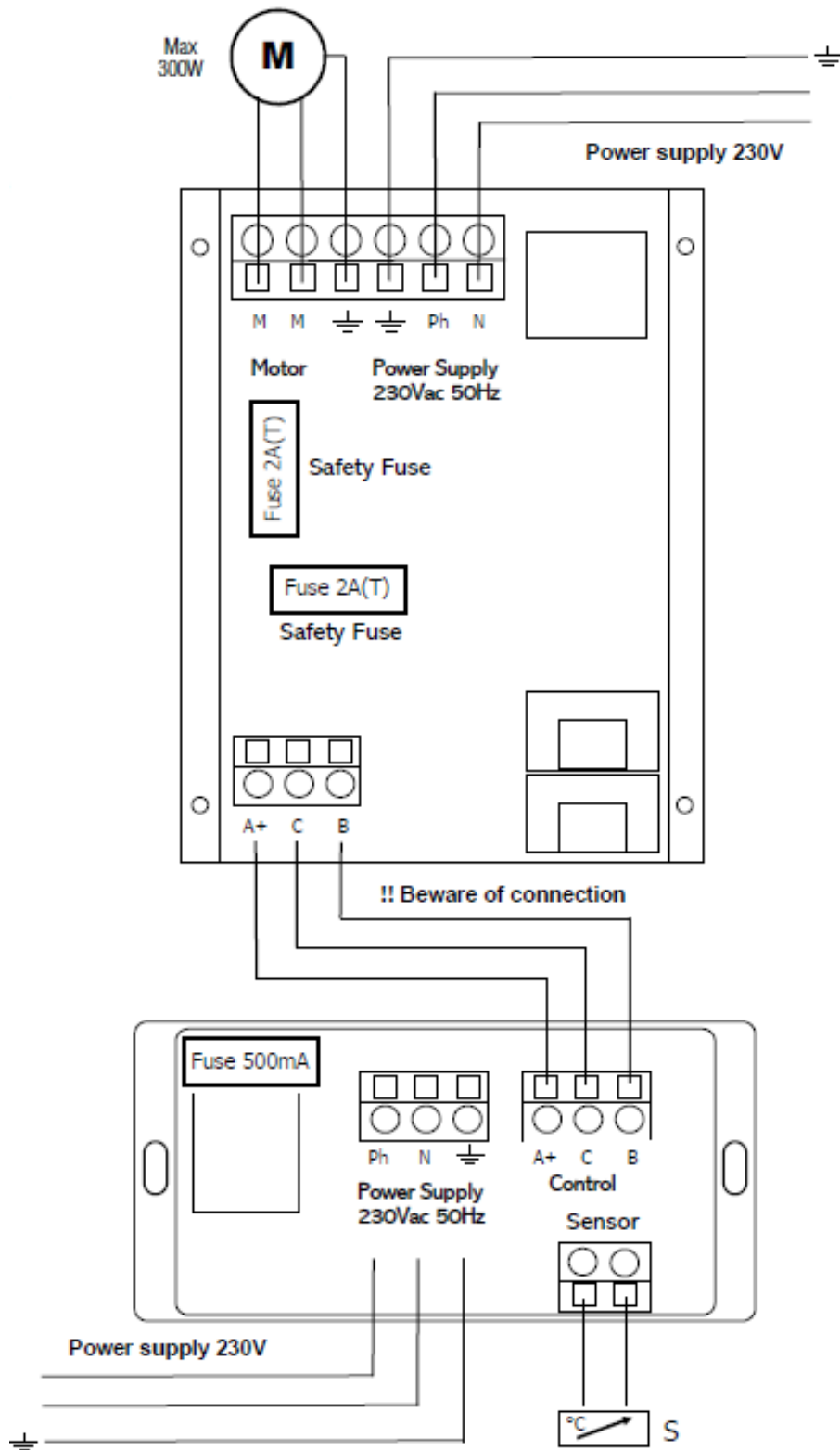
Figura nº17 - Conexões a serem feitas no controlador e no módulo de potência do Itaca eco C / V
